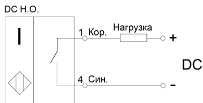
Рисунок 1 - Варианты схем подключения выключателей
