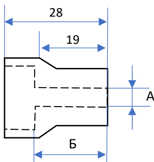
Рисунок 3 - Диафрагма ПВ-Д1-М18
