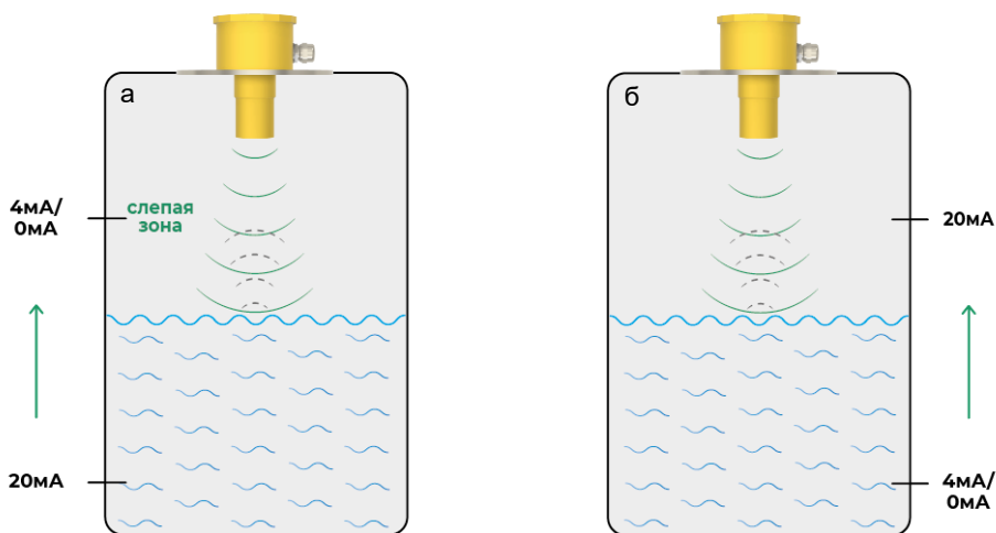
Рисунок 4 – Изменение тока аналогового выхода при наполнении (а – уменьшение, б – увеличение)
