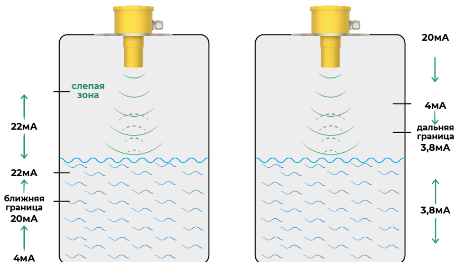
Рисунок 5 – Значения выходного тока в режиме 4-20мА за ближней или дальней границами, режим - увеличение тока при наполнении
