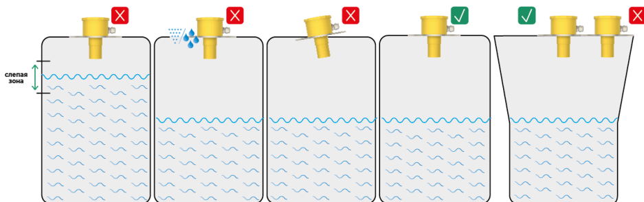
Рисунок 11 – Правила установки датчиков
