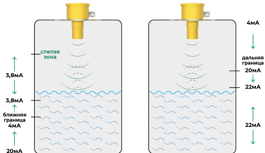
Рисунок 6 – Значения выходного тока в режиме 4-20мА за ближней или дальней границами, режим - уменьшение тока при наполнении
