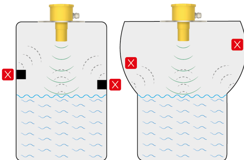
Рисунок 12 – Обнаружение датчиком сторонних\нежелательных объектов
