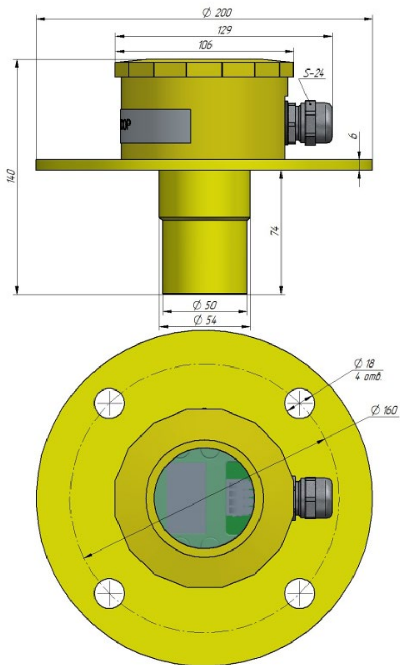
Рисунок 1 – Внешний вид датчика
