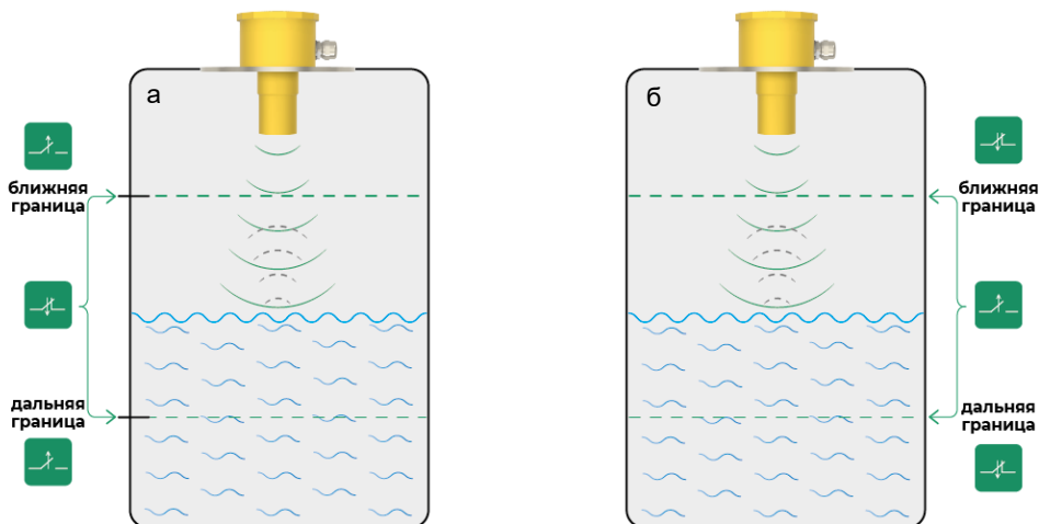
Рисунок 10 – Состояние дискретного выхода в режиме: а) «НО», б) «НЗ»
