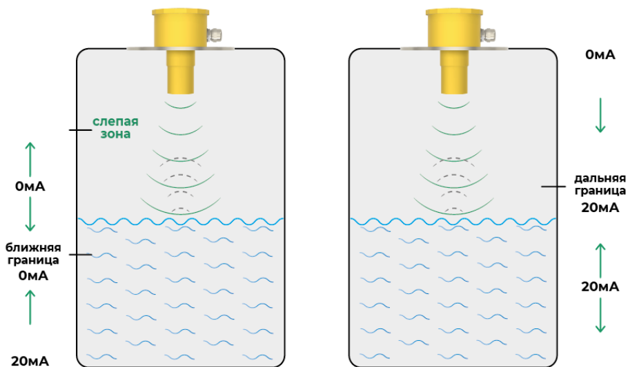
Рисунок 7 – Значения выходного тока в режиме 0-20mA за ближней или дальней границами, режим - уменьшение тока при наполнении
