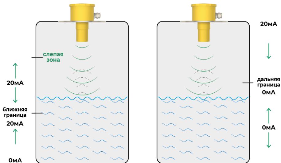
Рисунок 8 – Значения выходного тока в режиме 0-20mA за ближней или дальней границами, режим - увеличение тока при наполнении
