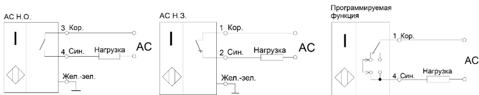
Рисунок 1 - Варианты схем подключения выключателей (цифрами указаны номера контактов клеммной коробки)
