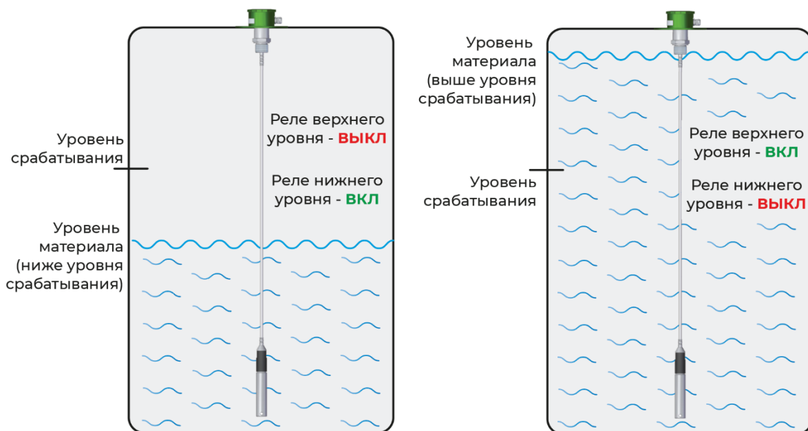
Рис.7 – Состояние реле P \uparrow и P \downarrow в однопороговом режиме
