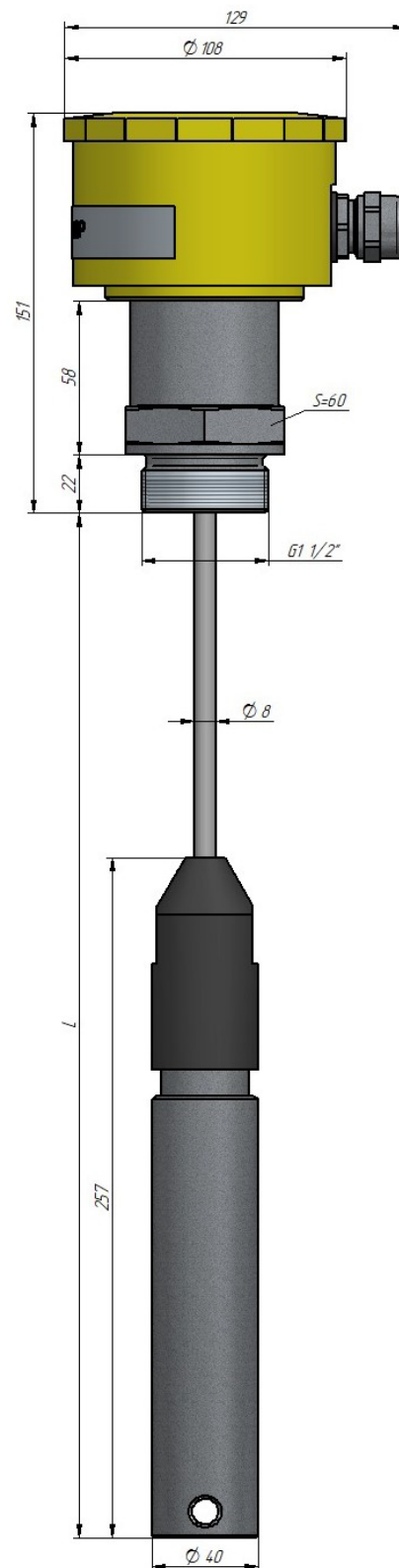
ДНЕ-хВ(020...-100)-117Кхх Рис. 1и. Изолированный гибкий ЧЭ для жидкости типа «В» без радиатора
