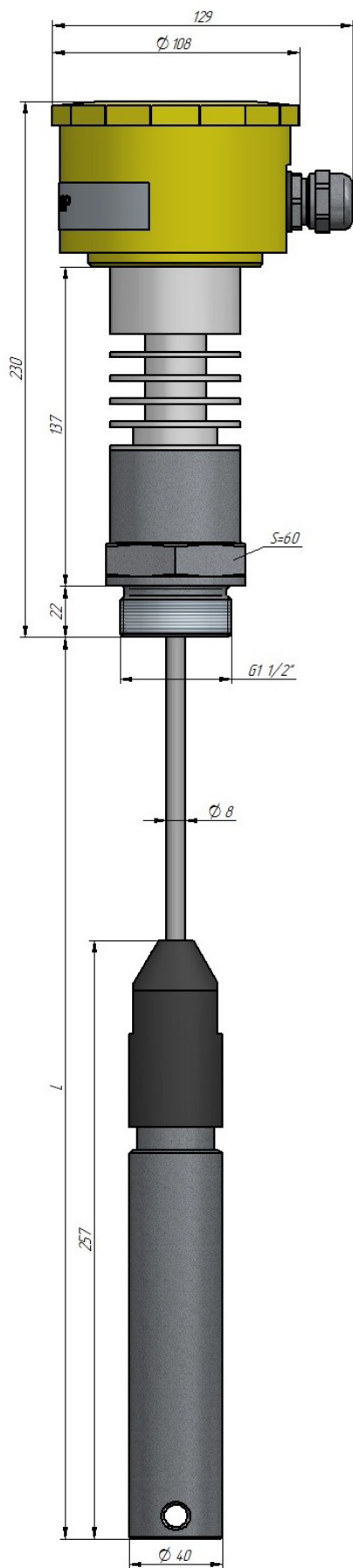
ДНЕ-хВ(02...100)-117Тхх Рис. 1з. Изолированный гибкий ЧЭ для жидкости типа «В» с радиатором
