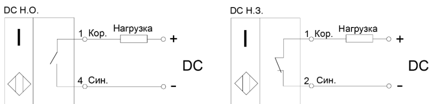
Рисунок 1 - Варианты схем подключения выключателей
