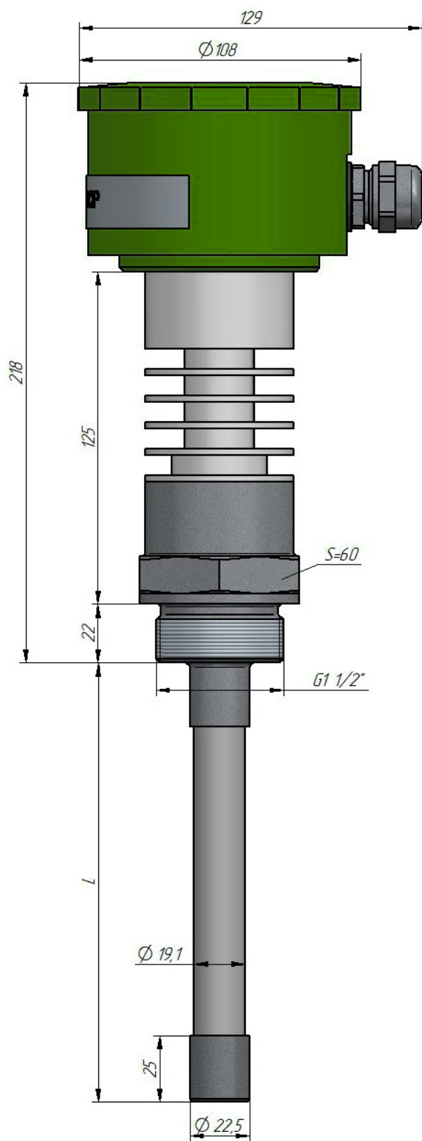
Рис. 16. Жесткий изолированный ЧЭ типа «Т» с радиатором
