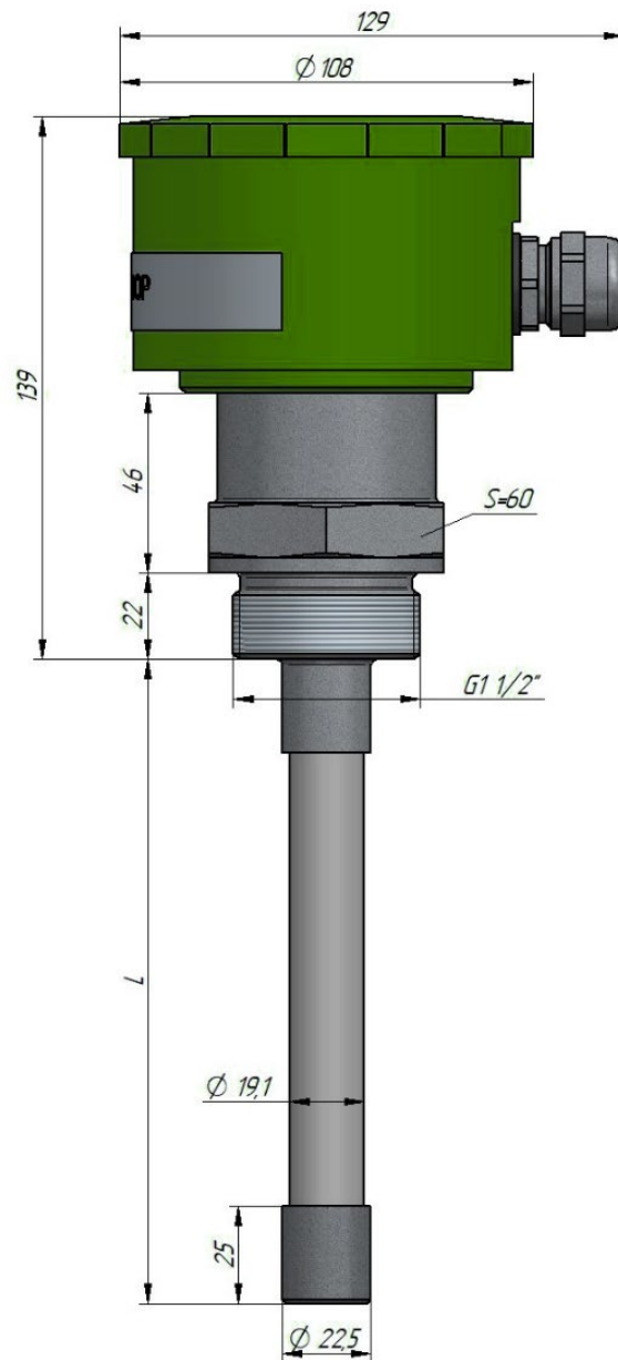
Рис. 1в. Жесткий изолированный ЧЭ типа «Т» без радиатора
