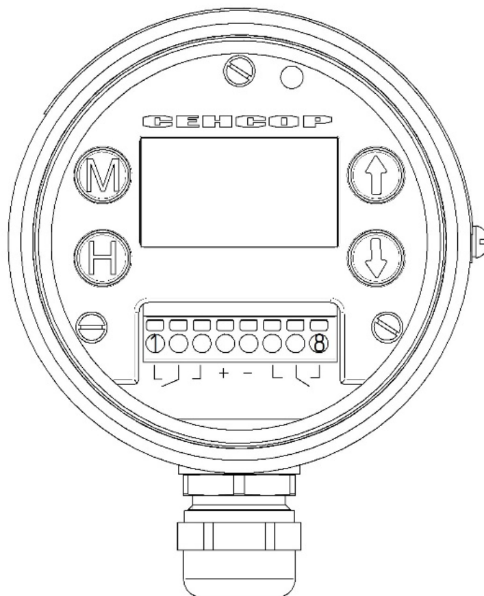
Рисунок 1а – Вид датчика изнутри
